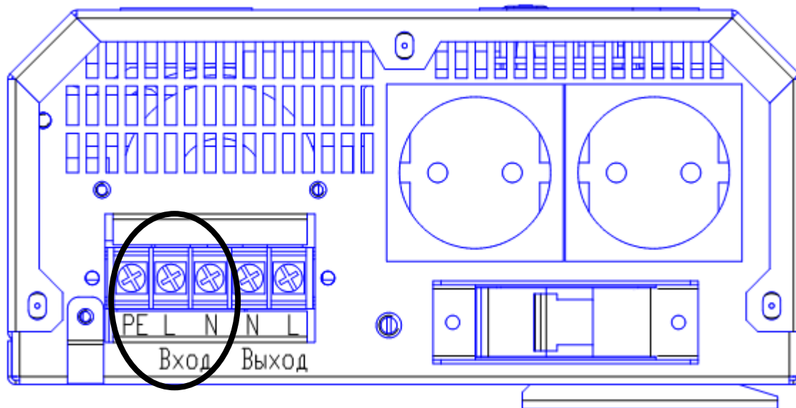
Рисунок 3.2 – Стабилизатор ИнСтаб IS2500 и ИнСтаб IS3500.
