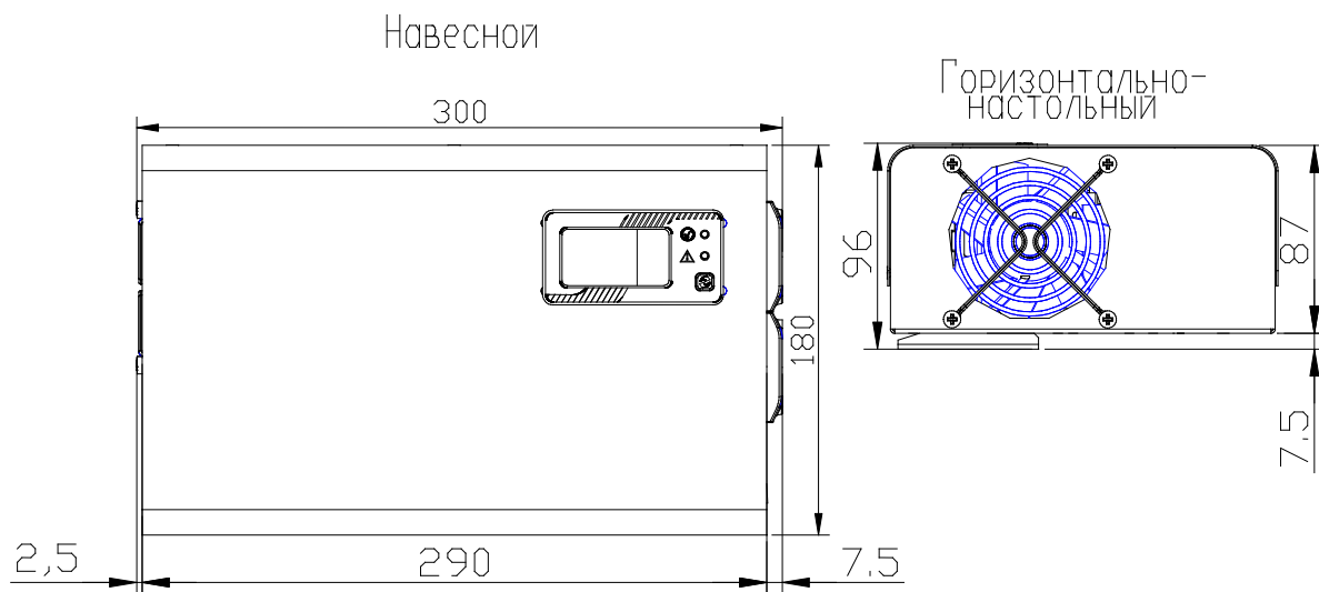
б) ИнСтаб IS1000; ИнСтаб IS1500
