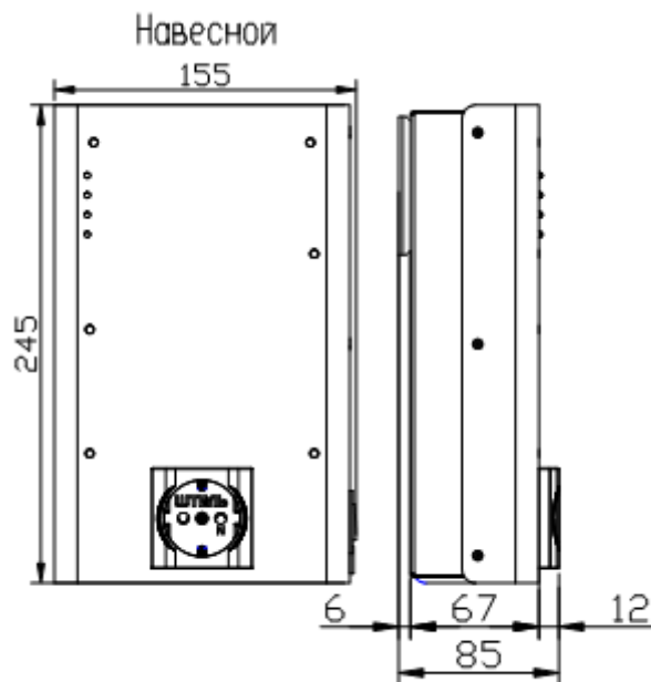
а) ИнСтаб IS350, ИнСтаб IS550
