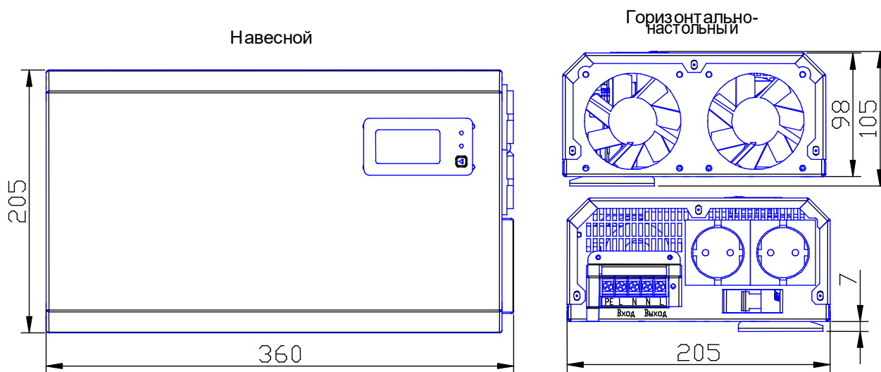
в) ИнСтаб IS2500, ИнСтаб IS3500
